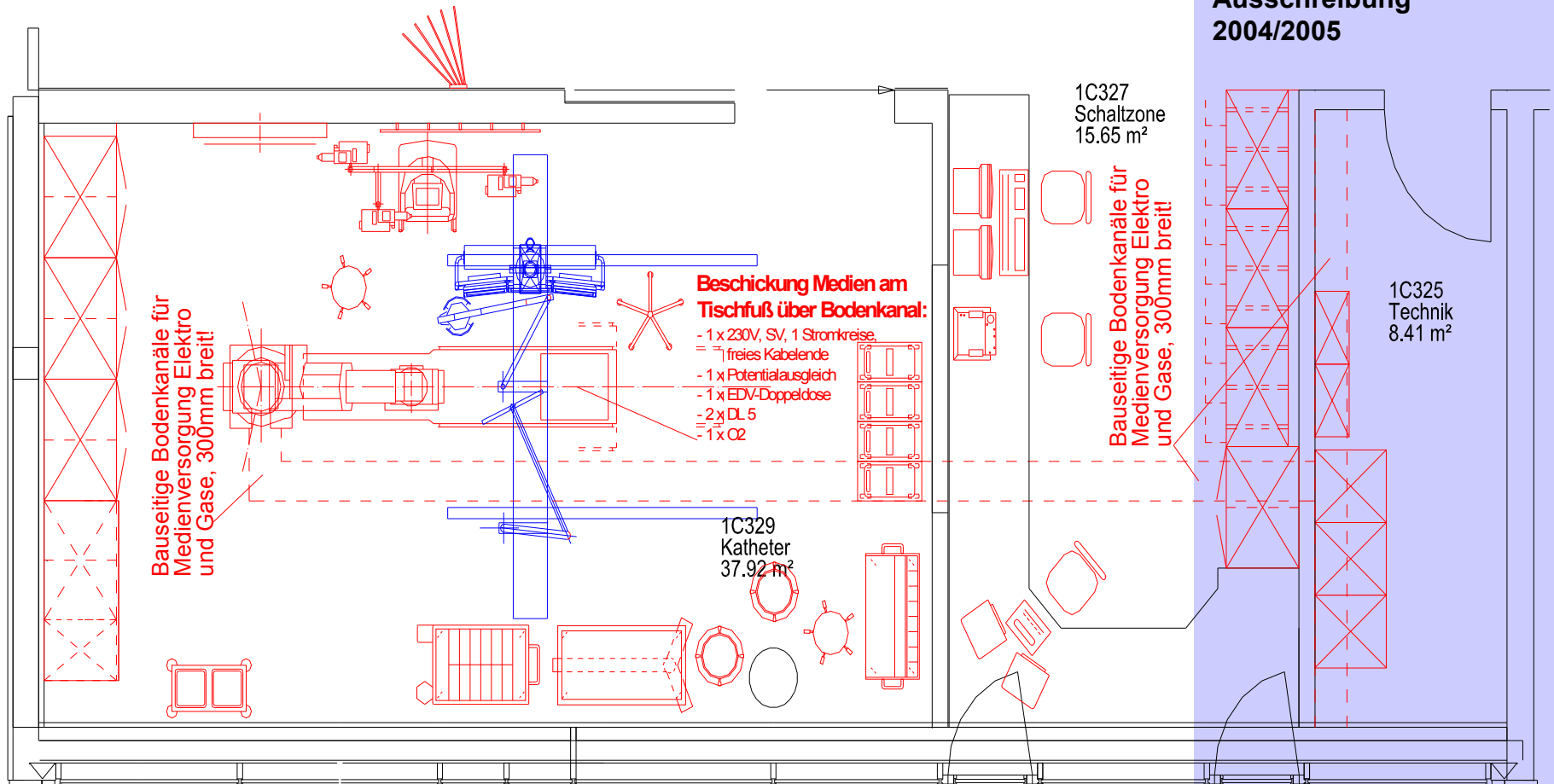
Ausschnittsvergrößerung eines Kathetermesslabors
